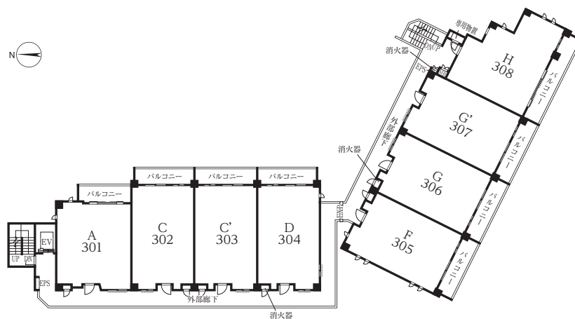
3 階平面図
