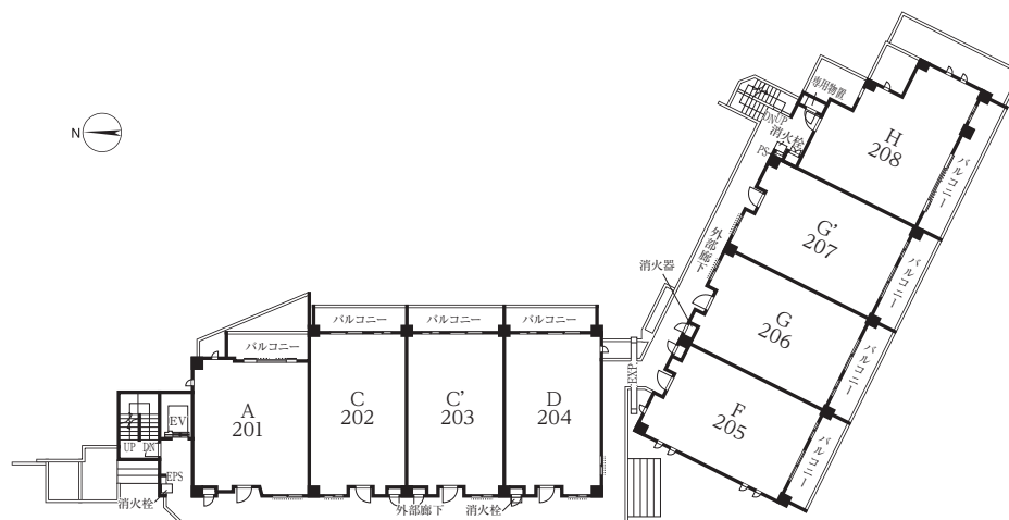
2 階平面図
